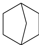
norbornane
